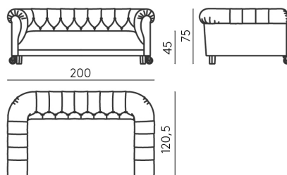
DIVANO L CM 200 _ CON RUOTE ANTERIORI _ PROFONDITA' CM 120,5 SOFA L CM 200_ WITH FRONT CASTORS_ DEPTH CM 120,5
