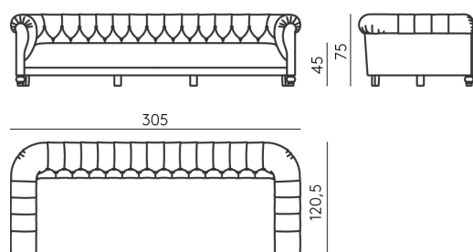
DIVANO L CM 305 _ CON PIEDINI ANTERIORI _ PROFONDITA' CM 120,5 SOFA L CM 305 _ WITH FRONT FEET _ DEPTH CM 120,5
