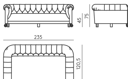
DIVANO L CM 235 _ CON RUOTE ANTERIORI _ PROFONDITA' CM 120,5 SOFA L CM 235 _ WITH FRONT CASTORS_ DEPTH CM 120,5
