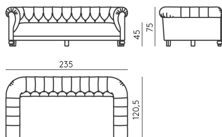
DIVANO L CM 235 _ CON PIEDINI ANTERIORI _ PROFONDITA' CM 120,5 SOFA L CM 235 _ WITH FRONT FEET _ DEPTH CM 120,5
