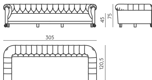
DIVANO L CM 305 _ CON RUOTE ANTERIORI _ PROFONDITA' CM 120,5 SOFA L CM 305 _ WITH FRONT CASTORS_ DEPTH CM 120,5
