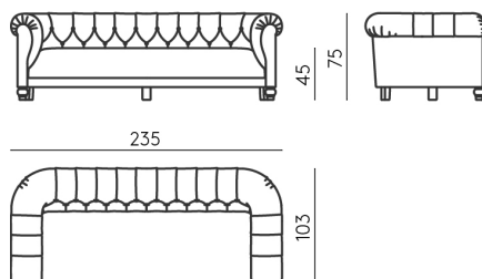
DIVANO L CM 235 _ CON PIEDINI ANTERIORI SOFA L CM 235 _ WITH FRONT FEET
