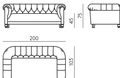
DIVANO L CM 200 _ CON PIEDINI ANTERIORI SOFA L CM 200 _ WITH FRONT FEET
